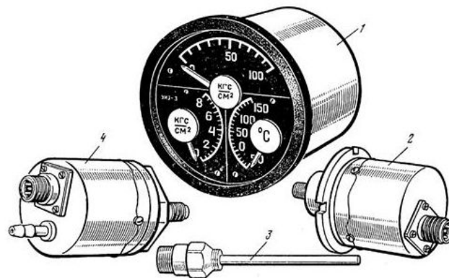
Рис. 2.36 - Комплект трехстрелочного моторного индикатора ЭМИ-3
