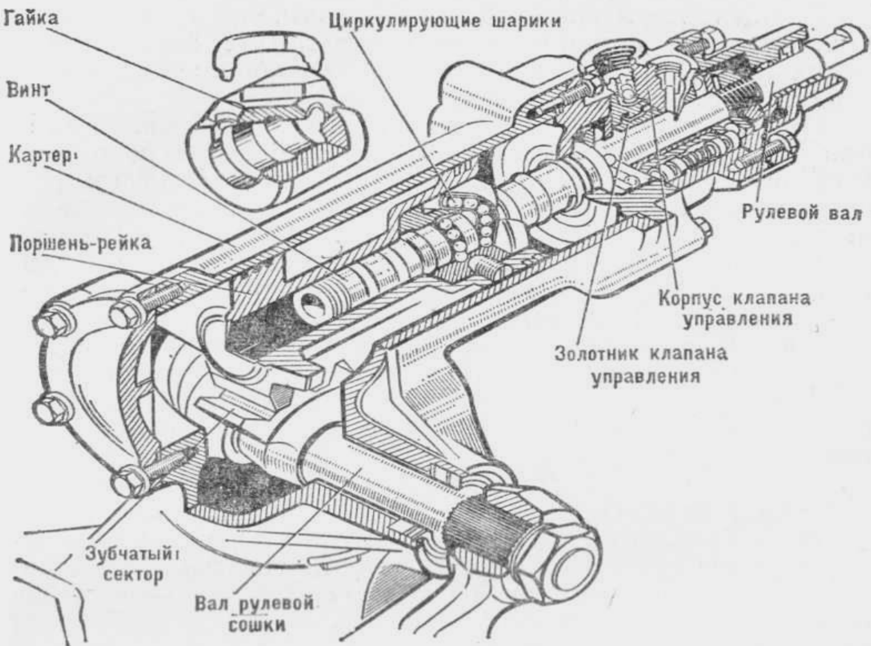
Рис. 160. Рулевой механизм автомобиля ЗИЛ-130
