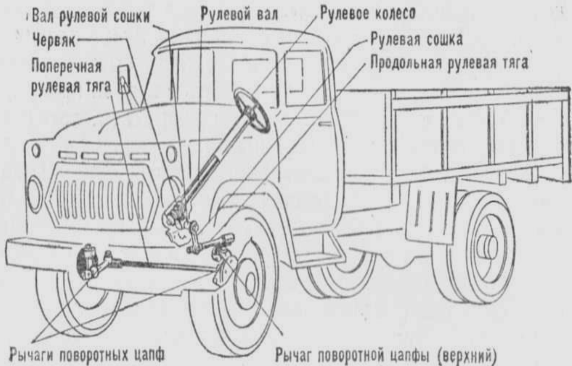
Рис. 158. Схема рулевого управления
