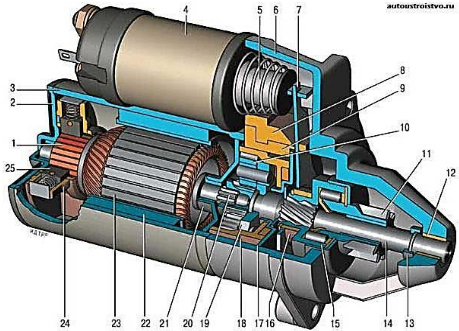
Схема стартера: 1 – коллектор; 2 – задняя крышка; 3 – корпус статора; 4 – тяговое реле; 5 – якорь реле; 6 – крышка со стороны привода; 7 – рычаг; 8 – кронштейн рычага; 9 – уплотнительная прокладка; 10 – планетарная шестерня; 11 – шестерня привода; 12 – вкладыш крышки; 13 – ограничительное кольцо; 14 – вал привода; 15 – обгонная муфта; 16 – поводковое кольцо; 17 – опора вала привода с вкладышем; 18 – шестерня с внутренним зацеплением; 19 – водило; 20 – центральная шестерня; 21 – опора вала якоря; 22 – постоянный магнит; 23 – якорь; 24 – щеткодержатель; 25 – щетка.
