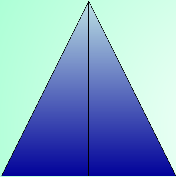
Равнобедренный треугольник
