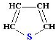
Тиофен
