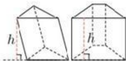
Призма
