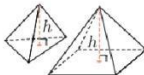
Пирамида
